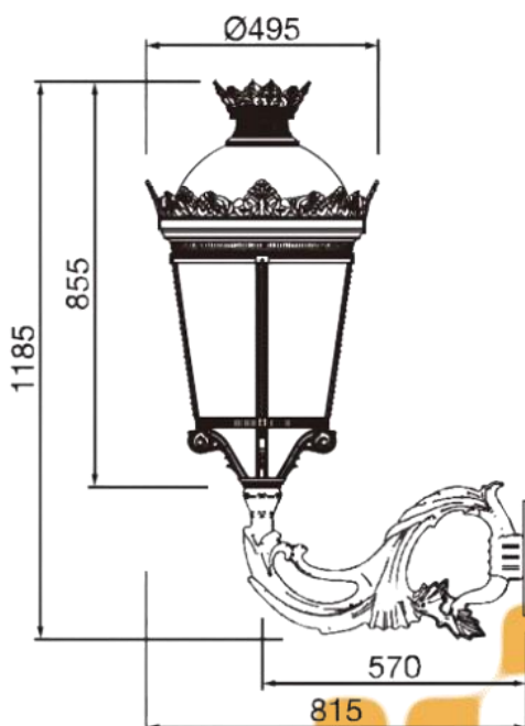
INSTALACIÓN LATERAL
